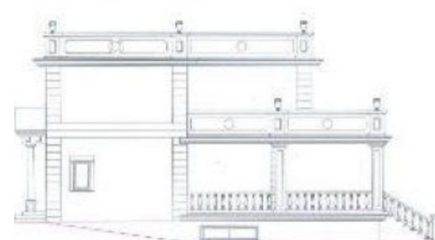
ALZADO SURESTE
